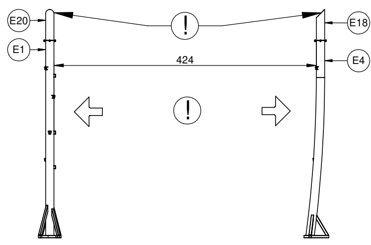
D-D (1 : 65)
